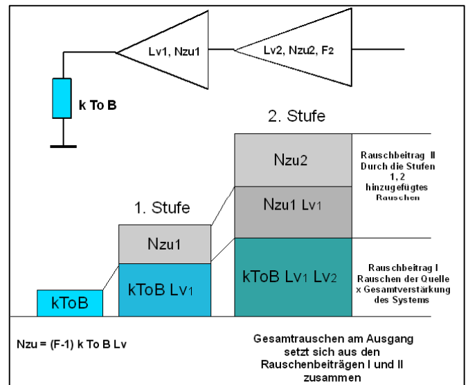
Bild 1. Rauschbeiträge einer 2 stufigen Anordnung rauschender Vierpole
