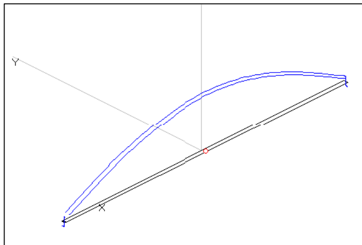
Bild 1: Stehende Welle auf dem Faltdipol bei Erregung in der Grundfrequenz f = 3,6 \text{ MHz}
