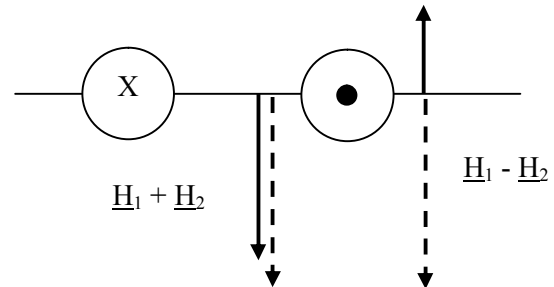
Bild 3: Magnetische Feldstärke zweier paralleler Leiter entgegengesetzter Stromrichtung, außerhalb der
