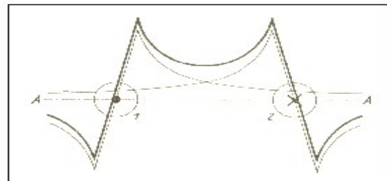
Bild 3: Magnetische Feldstärke zweier paralleler Leiter entgegengesetzter Stromrichtung, außerhalb der
